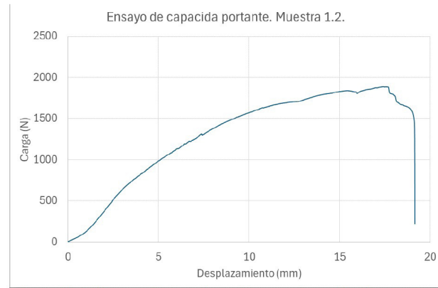
Gráfica carga desplazamiento del ensayo de tracción. Muestra 1.2.
