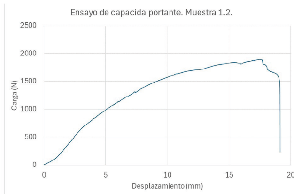
Figura nº 4. Gráfica carga desplazamiento del ensayo de tracción. Muestra 1.2.
